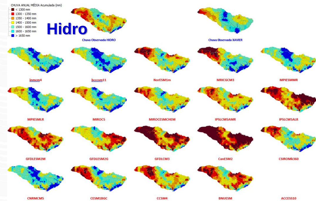
ura 5. Mapas de precipitação total anual observada (HIDRO e Xavier et al. (2015)) e estimada pelos 20 MCGs considerando o experimento RCP 8.5 (2011 a 2040).
