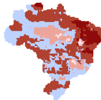
Intermediário (CCSM4-RCP8.5)
