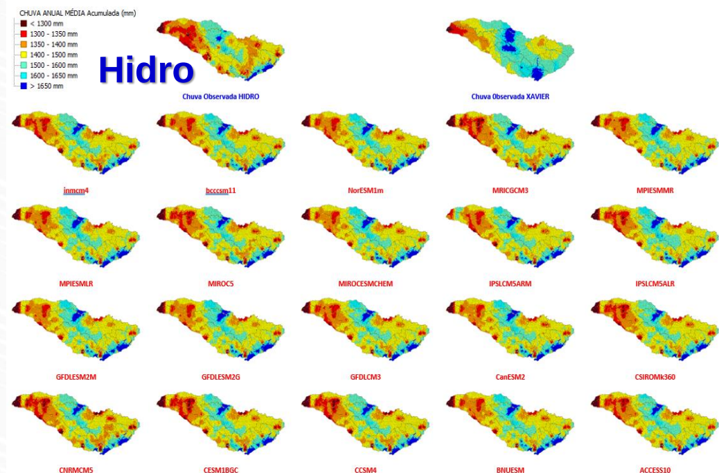
gura 1. Mapas de precipitação total anual observada (HIDRO e Xavier et al. (2015)) e estimada pelos 20 MCGs, considerando o experimento Historical (1950 a 2005).
